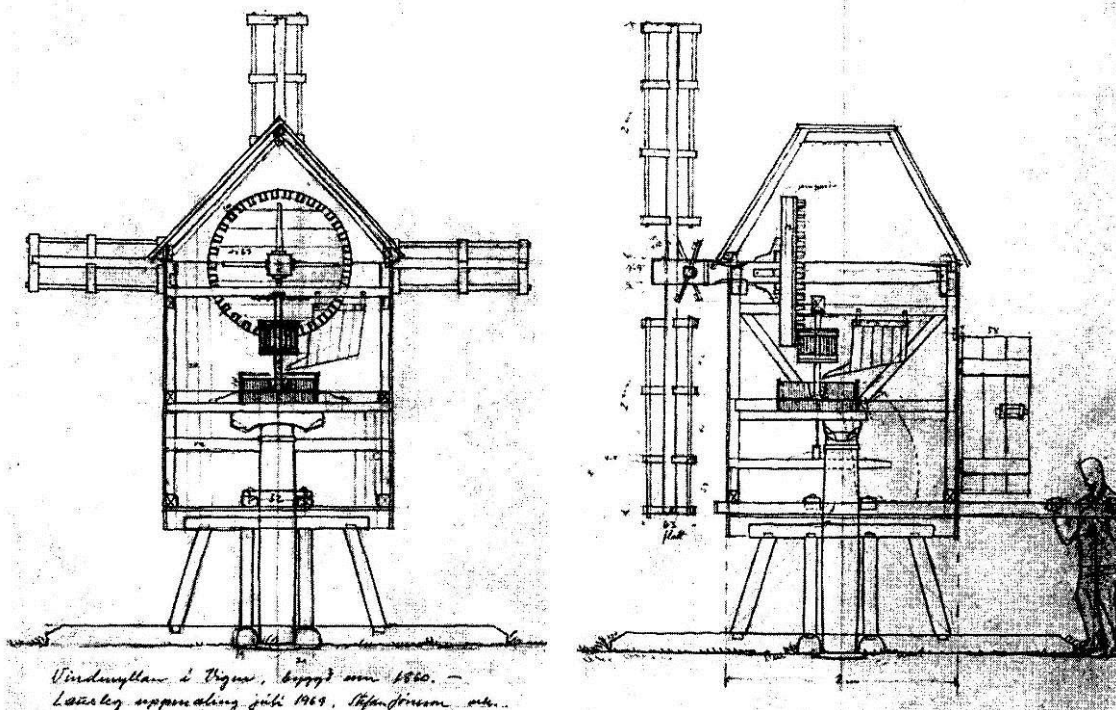
Vindmyllan í Vigur, skurðmyndir. Teikningar Stefáns Jónssonar arkitekts.
