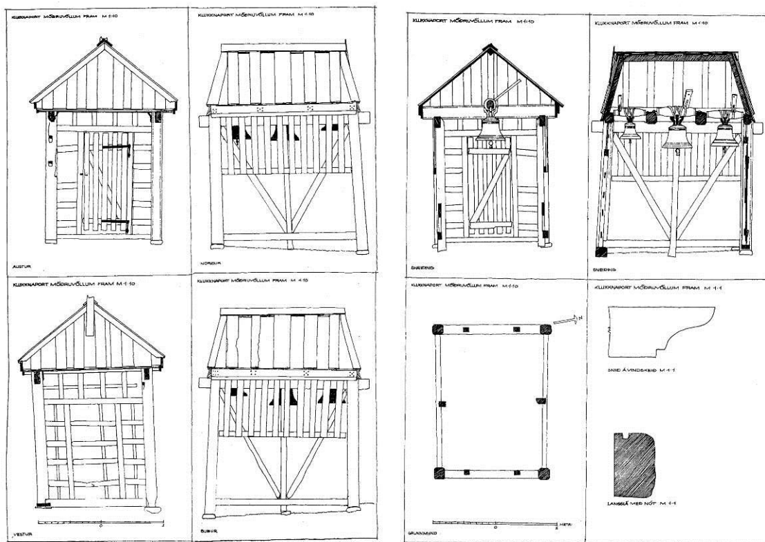
Klukknaportið á Möðruvöllum, útlit, skurðmyndir, grunnmund og deili. Teikningar Harðar Ágústssonar.
